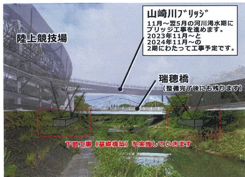
山崎川ブリッジ 下部工事
