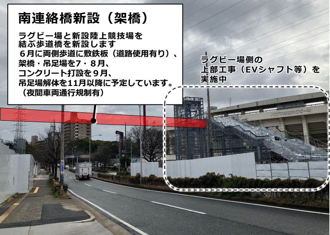
南連絡橋新設 上部工事
